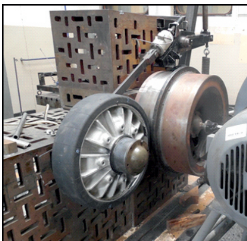
zkoušky pojezdových kol pásových vozidel
