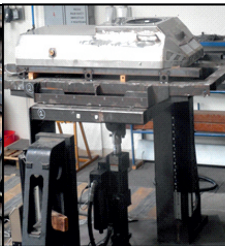
zkoušky mechanické odolnosti klimatizací
