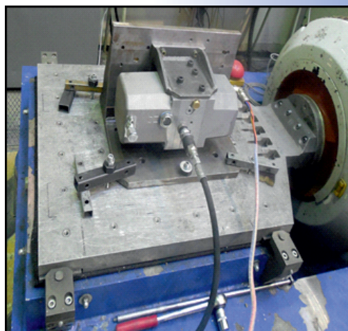
zkoušky mechanické odolnosti brzdových systémů kolejových vozidel
