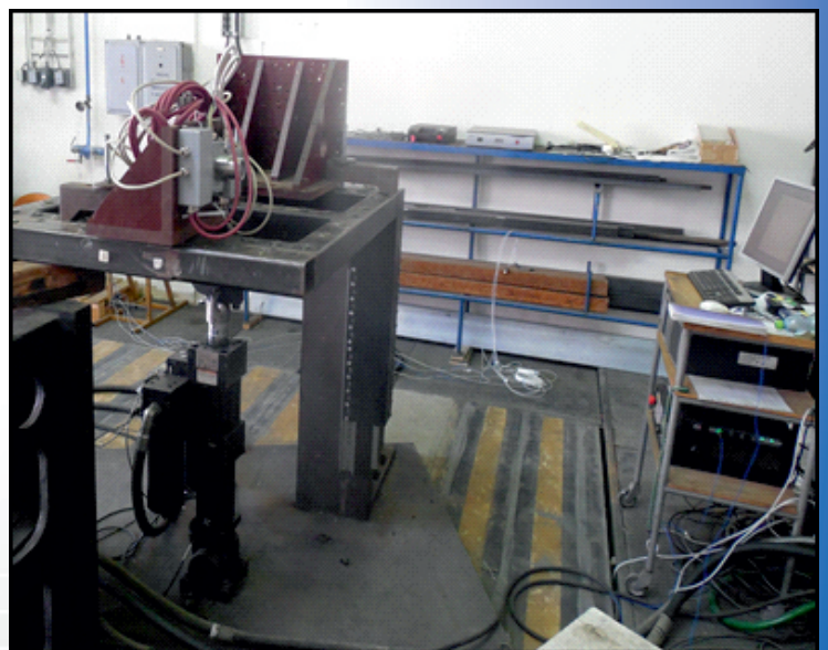
seizmické způsobilosti technologií jaderných elektráren-stend MTS (záložní AKB)
