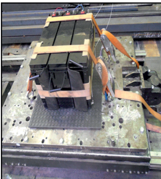
seizmické způsobilosti technologií jaderných elektráren-stend MTS (záložní AKB)
