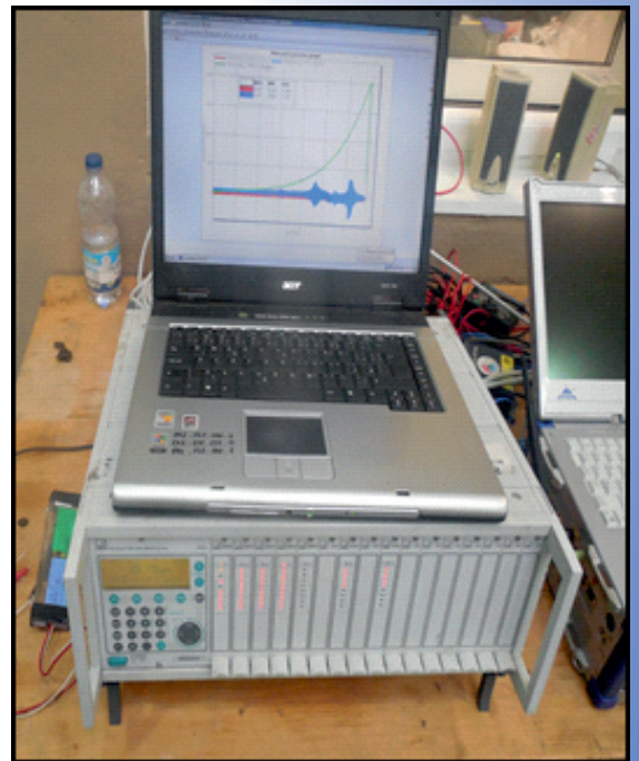
fyzikálních veličin měřicí ústředna HBM MGCplus
