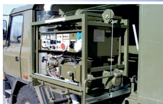
Výsuvná klec s EC vně schrány
