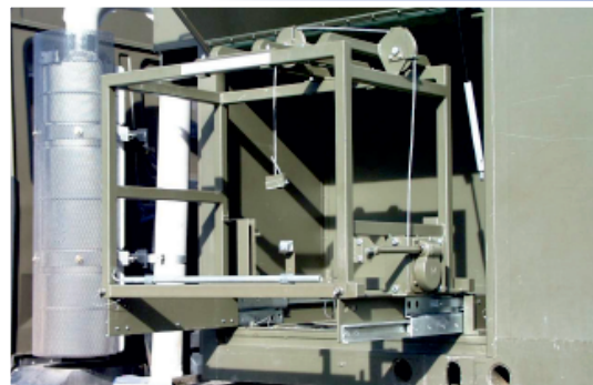
Výsuvná klec bez EC vně schrány
